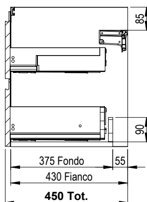
SEZIONE A-A
