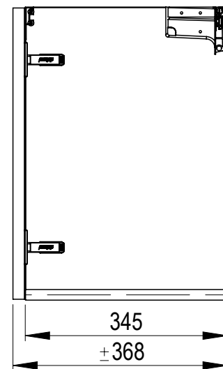
SEZIONE A-A
